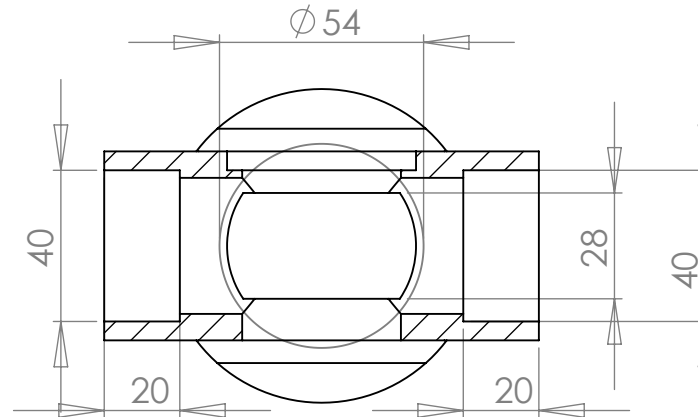
COUPE B-B
